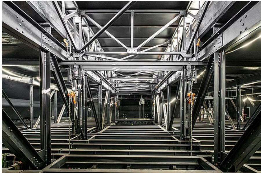
Abbildung 6: Bühnentechnik des Schnürbodens nach dem Umbau. Quelle: Maren Szech, VCC
